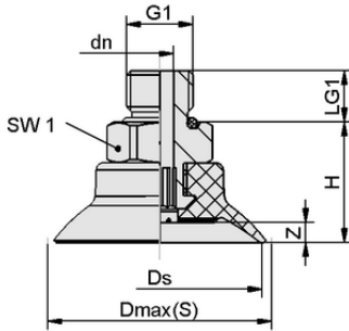
Tasarım verileri SUF 20 HT1-60 G1/8-AG
