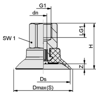
デザインデータ SUF 25 NBR-ESD-55 G1/8-IG
