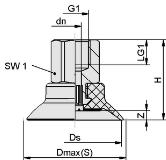
デザインデータ SUF 18 NBR-55 G1/8-IG
