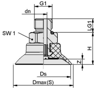
Tasarım verileri SUF 15 NBR-55 G1/8-AG
