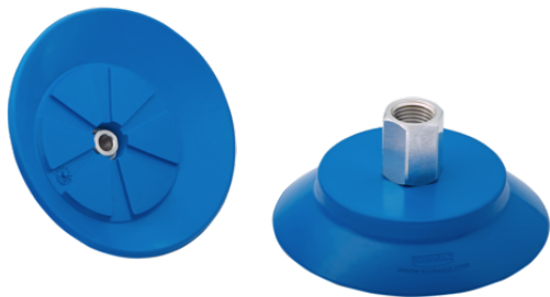
SUF 80 HT1-60 G1/4-IG
