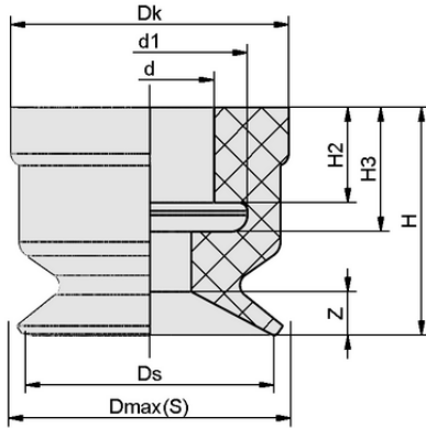
Tasarım verileri SUF 8 NBR-ESD-55 SC020
