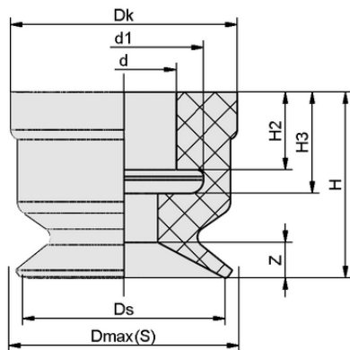
Datos de diseño SUF 8 NBR-ESD-55 SC020
