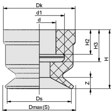
Données de construction SUF 8 NBR-ESD-55 SC020
