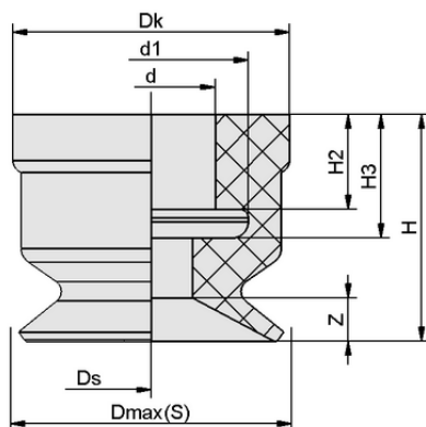
デザインデータ SUF 6 SI-CO-55 SC020
