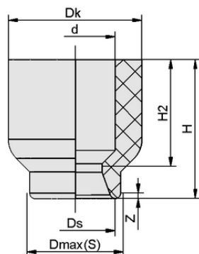
Datos de diseño SUF 2 NBR-ESD-55 SC010
