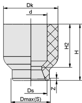
Конструктивные данные SUF 1.5 NBR-ESD-55 SC010
