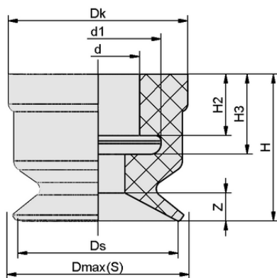
Dati di costruzione SUF 5 HT1-60 SC020
