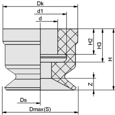
Tasarım verileri SUF 8 SI-55 SC020
