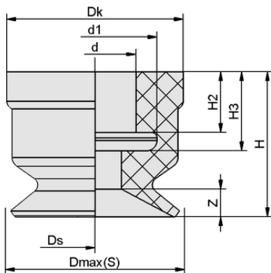
Datos de diseño SUF 6 SI-55 SC020
