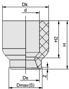
Datos de diseño SUF 1.5 SI-55 SC010
