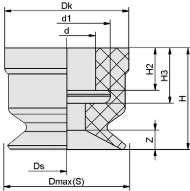
Tasarım verileri SUF 6 NBR-55 SC020
