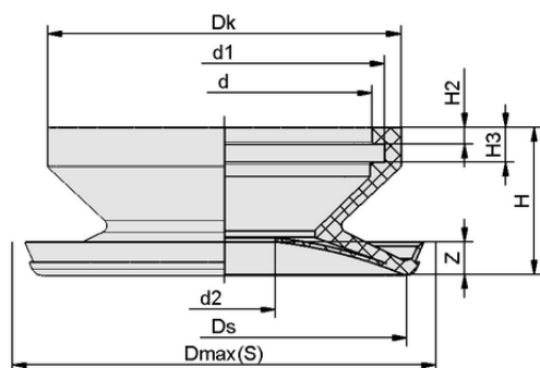
デザインデータ SPL-HT 120 FPM-F-65
