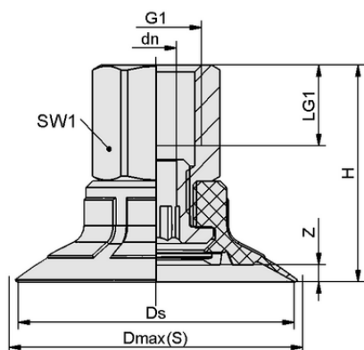
デザインデータ SPF 60 ED-65 G1/4-IG
