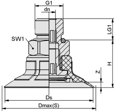
Tasarım verileri SPF 50 ED-65 G1/4-AG
