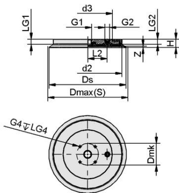
Datos de diseño SGF 125 HT1-60 G3/8-IG
