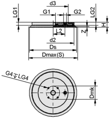
Tasarım verileri SGF 125 HT1-60 G3/8-IG
