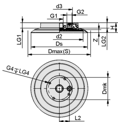
Конструктивные данные SGF-HS 150 HT1-60 G1/2-IG
