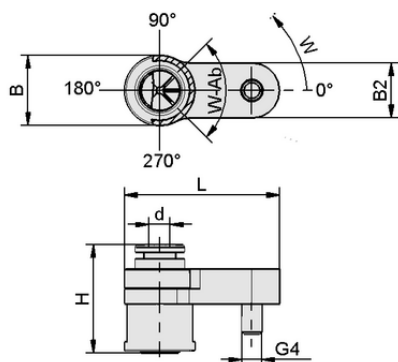
Конструктивные данные SBSm 14 90-3 4/2 90
