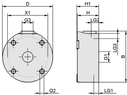
Dati di costruzione SBS 120 SF G1/8-IG AL
