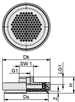
Конструктивные данные SPL 115 POM-NBR G1/4-IG
