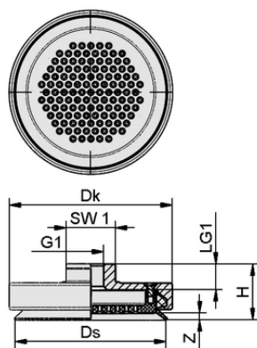
デザインデータ SPL 70 POM-NBR G1/4-IG
