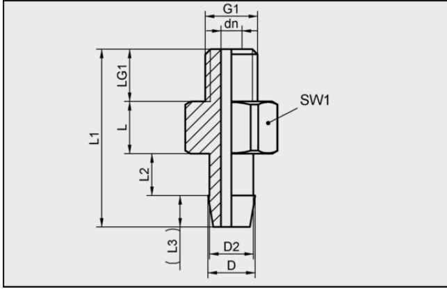
Tasarım verileri SA-NIP N055 M5-AG DN100
