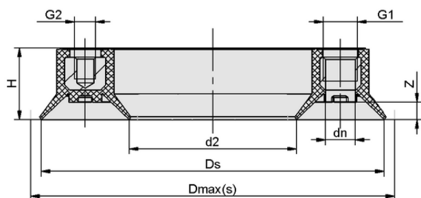
Konstruktionsdaten SR-DBD 130 NBR-60
