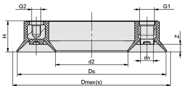
Datos de diseño SR-DBD 130 NBR-60
