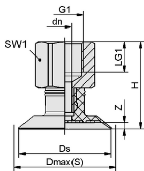
Dati di costruzione SGPN 20 FPM-65 G1/8-IG
