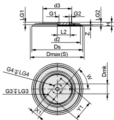
Конструктивные данные SGF-HS 350 EPDM-55 G1/2-IG
