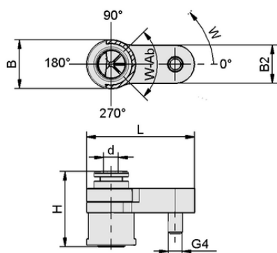
Конструктивные данные SBSm 14 90-3 4/2 0
