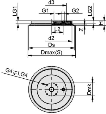
Tasarım verileri SGF 125 HT1-60 G1/4-IG
