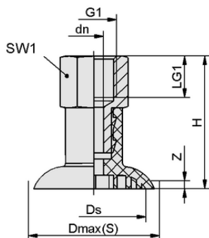
Конструктивные данные SGPN 35 HT1-60 G1/4-IG
