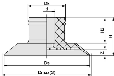
Datos de diseño SGP 40 HT1-60 N035
