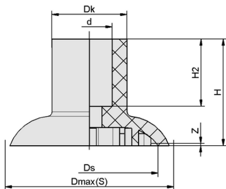
Datos de diseño SGP 35 HT1-60 N034
