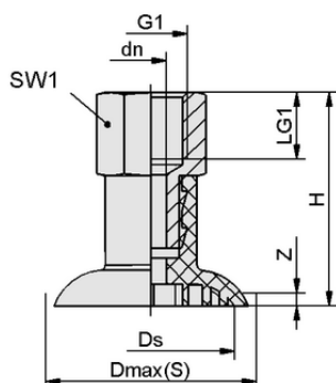
Конструктивные данные SGPN 35 SI-50 G1/4-IG
