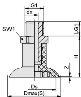
Конструктивные данные SGPN 35 SI-50 G1/4-AG
