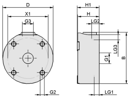
Dati di costruzione SBS 40 SF G1/8-IG CS AL
