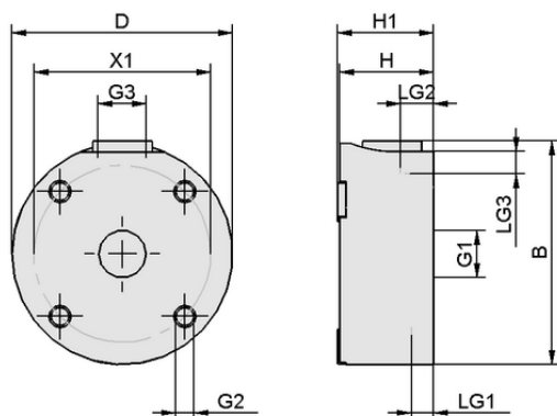
Конструктивные данные SBS 20 HF M5-IG AL
