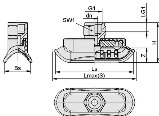
デザインデータ SAOK 70x25 NBR-60 G1/4-IG
