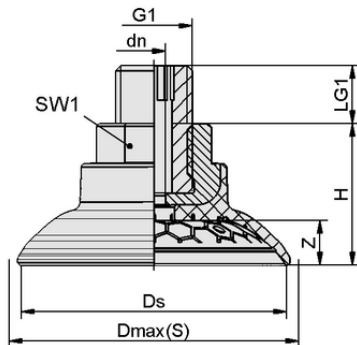
Dati di costruzione SAG 45 NBR-60 M10-AG
