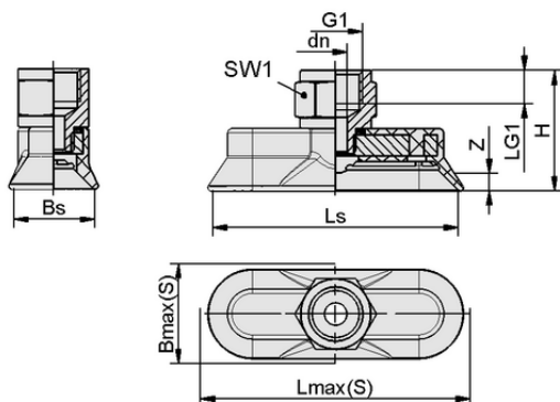
Dati di costruzione SAOG-S 80x30 NBR-60 G1/4-IG
