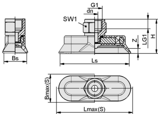
Données de construction SAOG-S 80x30 NBR-60 G1/4-IG
