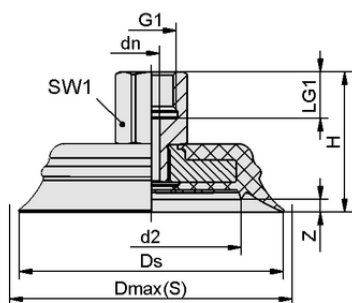
デザインデータ SHFN 70 NK-45 G1/4-IG E
