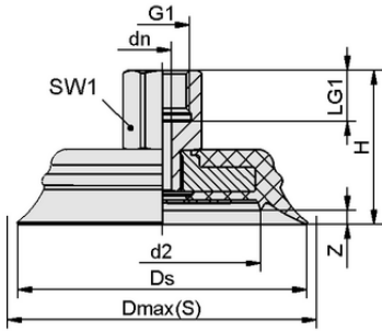
Tasarım verileri SHFN 70 NK-45 G1/4-IG E
