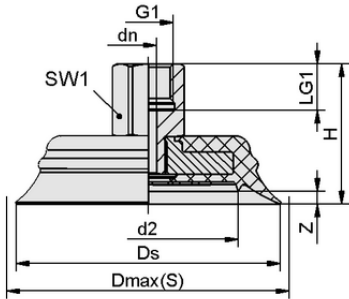
Tasarım verileri SHFN 85 NK-45 G1/4-IG E
