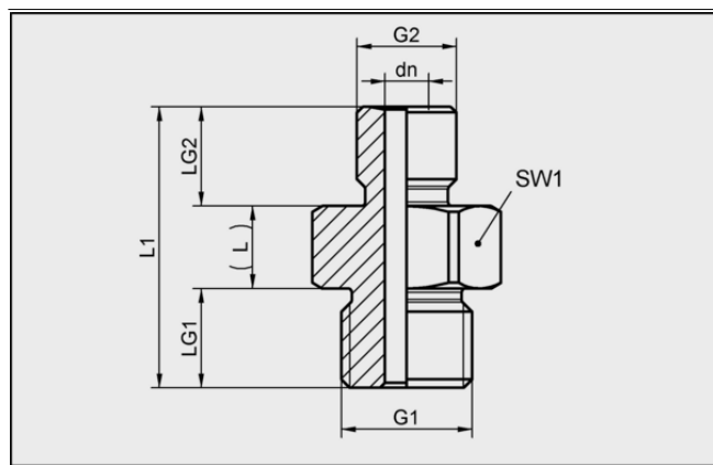
Datos de diseño RED-NIP G1/4-AG M10x1.25-AG AL
