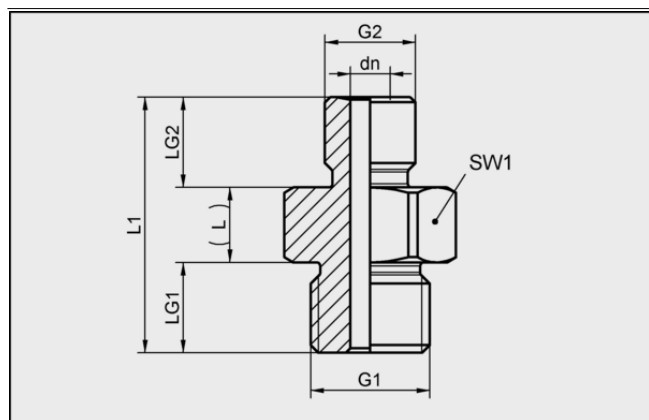
Конструктивные данные RED-NIP G1/4-AG M10x1.25-AG AL
