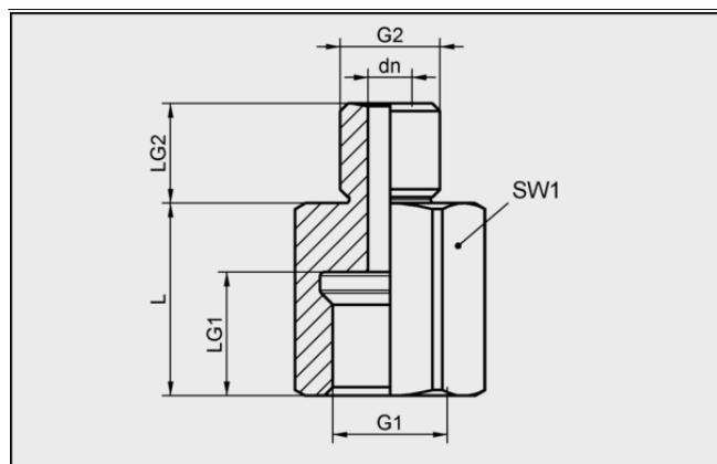
Datos de diseño SA-NIP N009 G1/4-IG DN440
